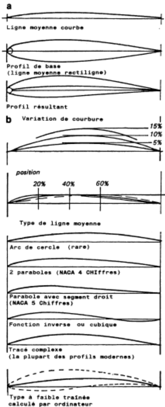
Figure 3.9 : géométrie de base des profils. Cliché MRA.
